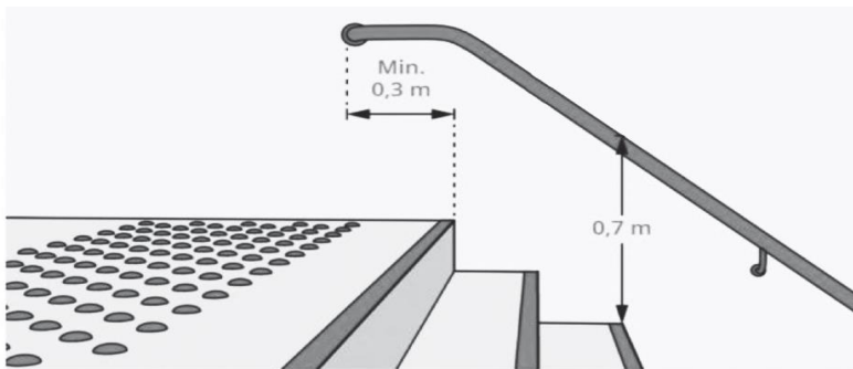
§ 12-14 Figur 2. Enten kan én håndløper monteres med overkant 0,9 meter over forkanten på innterrnet og med den andre 0,2 meter lavere, eller én håndløper kan monteres i 0,8 meter høyde.
