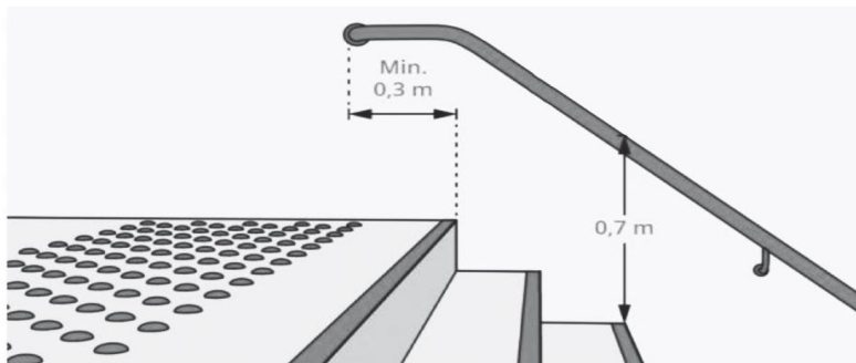
§ 12-14 Figur 2. Enten kan én håndløper monteres med overkant 0,9 meter over forkanten på inntretnet og med og den andre 0,2 meter lavere, eller én håndløper kan monteres i 0,8 meter høyde.
